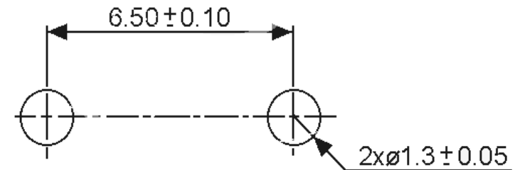
P.C.B. Layout
