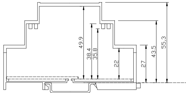
BARRA DIN
