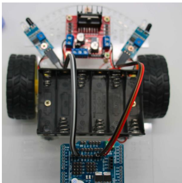
Figure 8 - 2 : Emplacement de chaque capteur avec le module Shield. Attention à la polarité.
