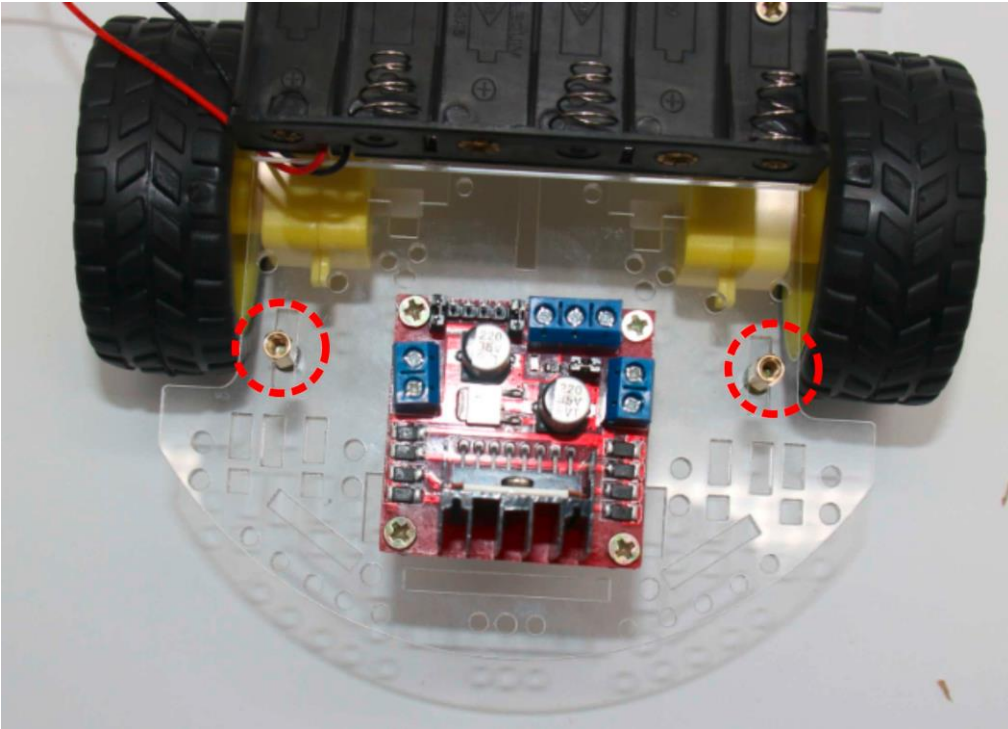
Figure 6-2 : Installation des deux séparateurs à l'aide de vis M3 x 10mm.
