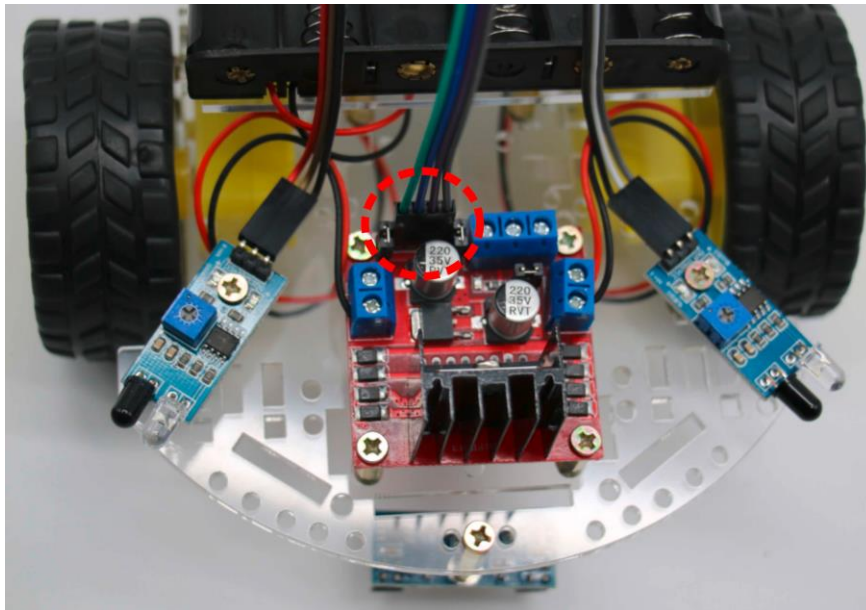
Figure 8 – 3 : Emplacement de l'alimentation des moteurs
