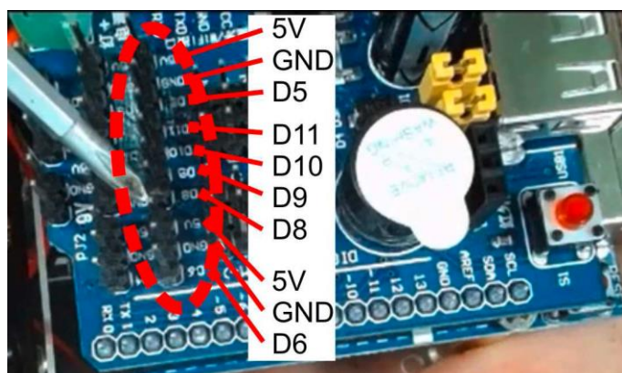
Figure 8 – 1 : Emplacement des contacts sur le module Shield
