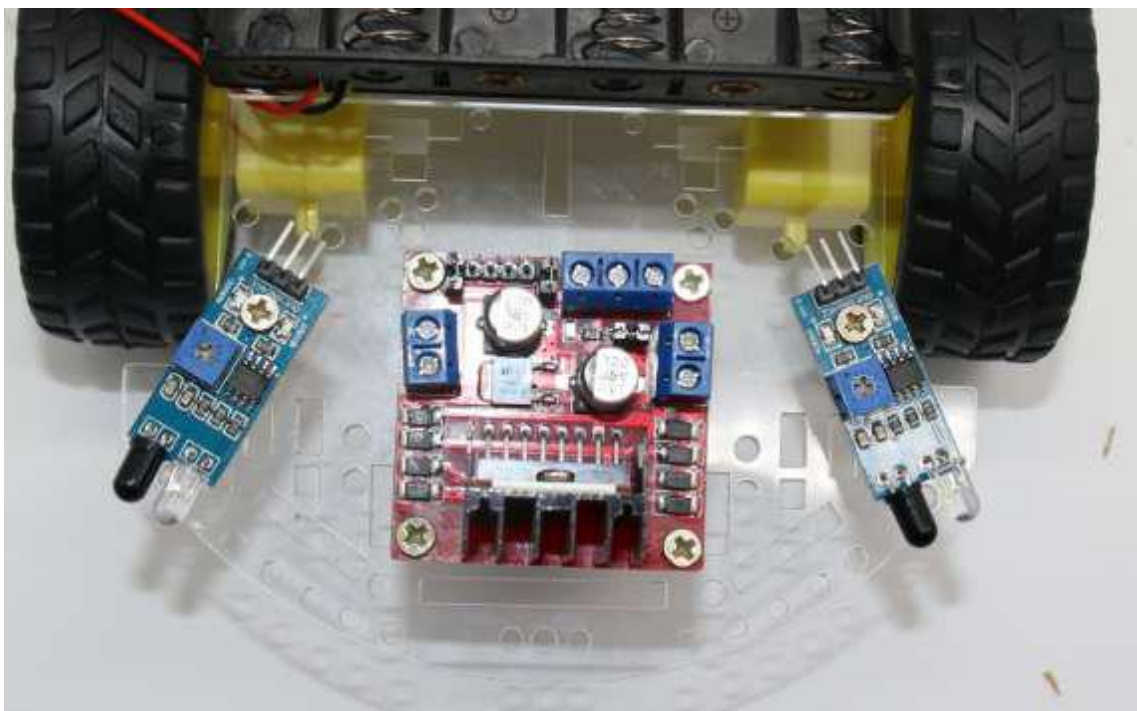
Figure 6-3 : Modules IR pour éviter les objets fixés à l'aide de vis M3 x 8mm. Fixer les deux capteurs dans la même position que l'image.
