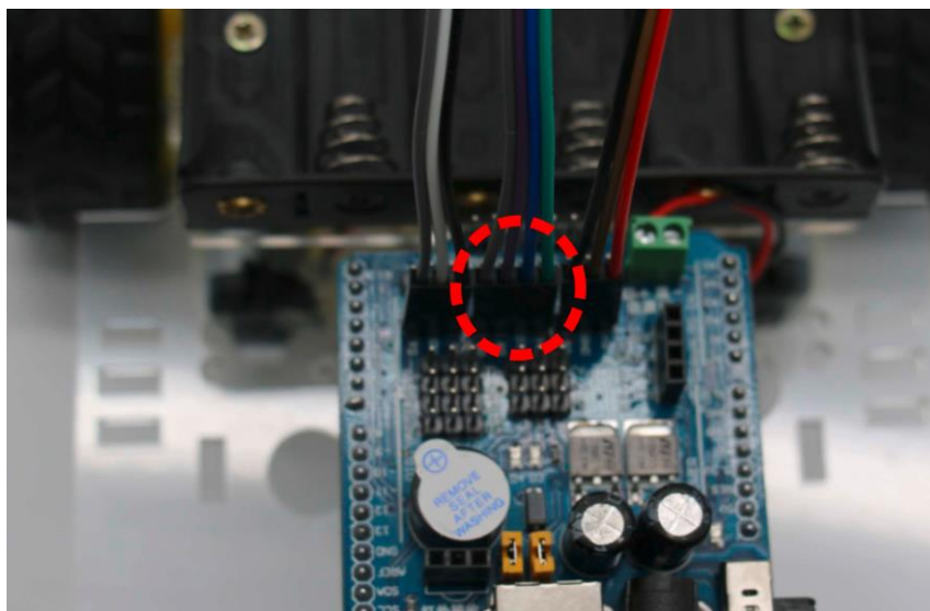
Figure 8 – 4 : Vue de l'autre extrémité des câbles connectés au module Shield. Attention à la polarité selon le tableau suivant. Il est préférable de passer ce câble entre le porte piles et le châssis acrylique.
